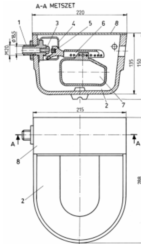
6. ábra: Úszószelepes szintszabályozós önitató
