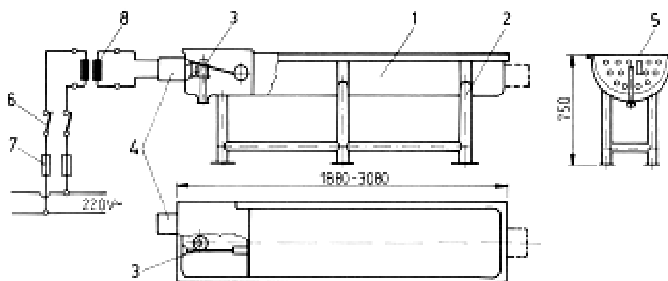
11. ábra: Temperált vizű önitató vályú
